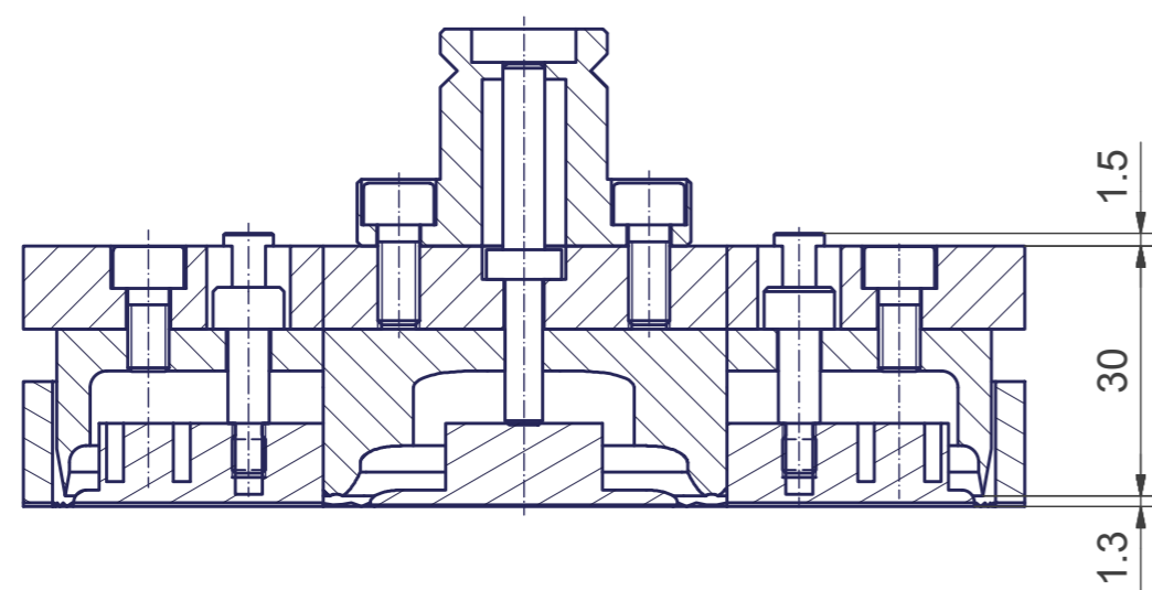
A-A (1:1)
