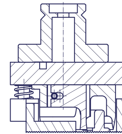
A-A (1:1)
